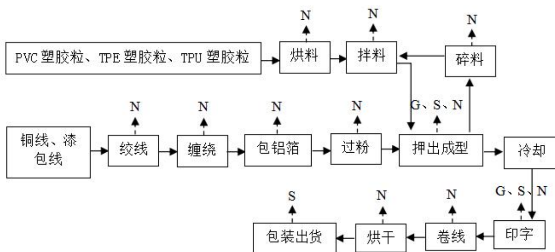
图 3-3 项目生产工艺及产污环节流程图
